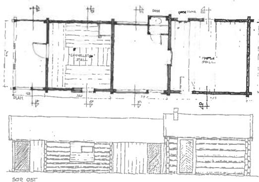
Oppmåling 1979 av Gammelstua og Nystua i Kvænangsbott. Arkitekt MNAL Petter Bakke
