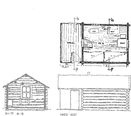
Oppmåling 1979 av Dalstua
